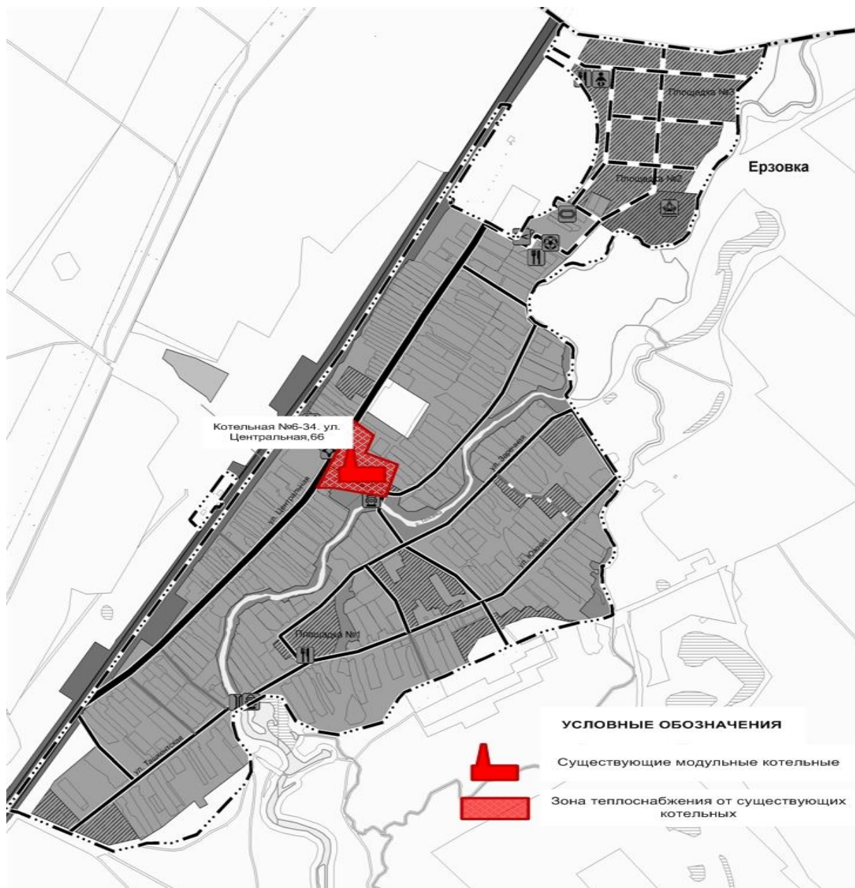
Рисунок 1.12.5.1– Источники тепловой энергии с. Ерзовка
