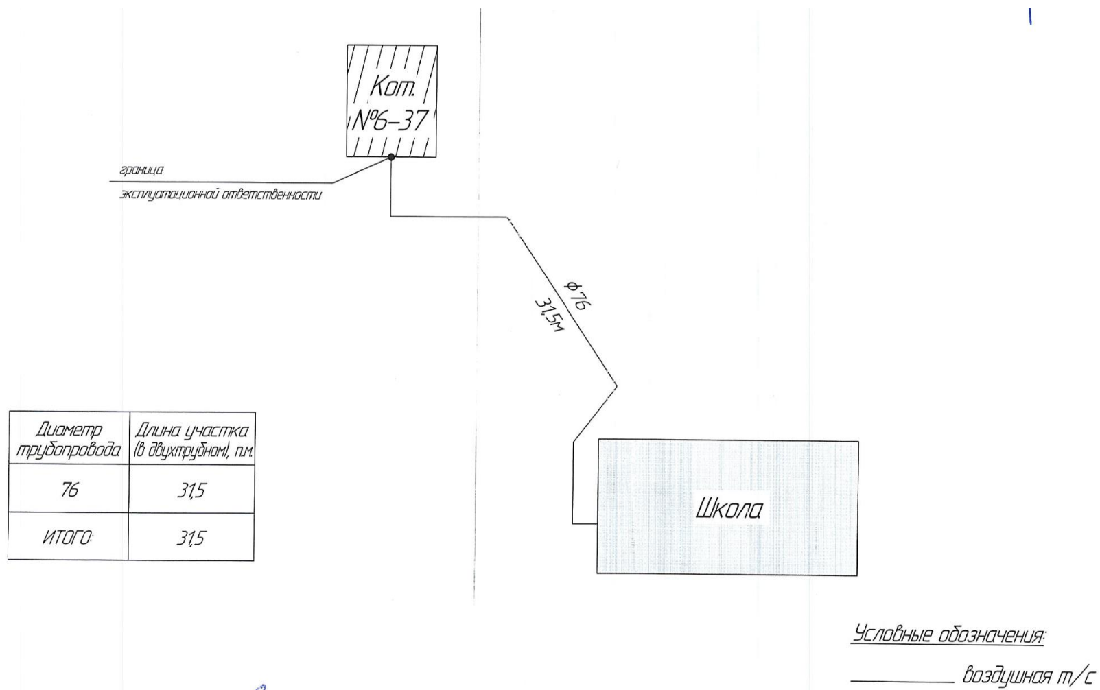
Рисунок 1.3.2.3 – Схема тепловых сетей котельной №6-37 п. Вязники
