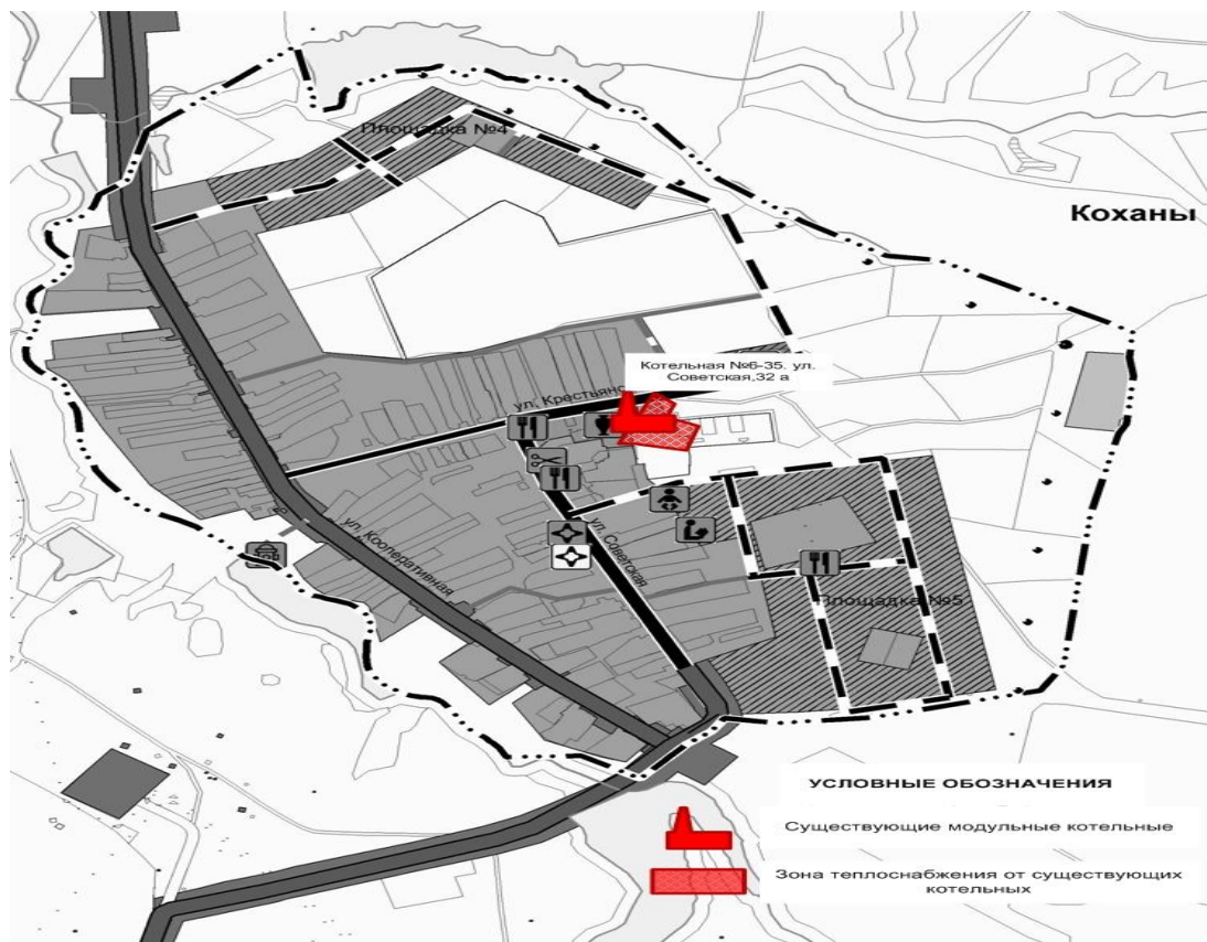
Рисунок 1.4.1 - Зоны действия модульной котельной с. Ерзовка
