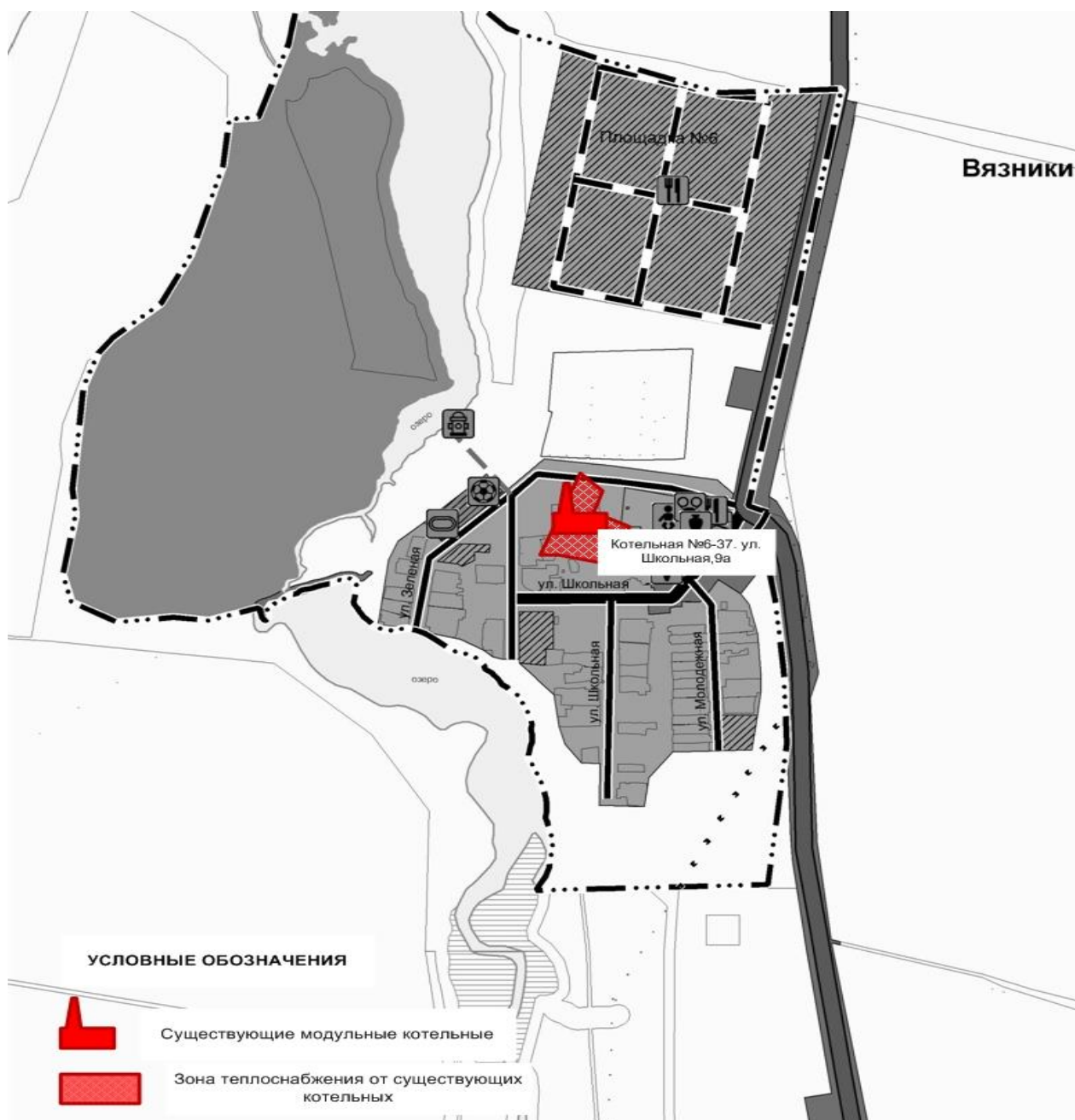
Рисунок 1.12.5.2– Источники тепловой энергии п. Вязники
