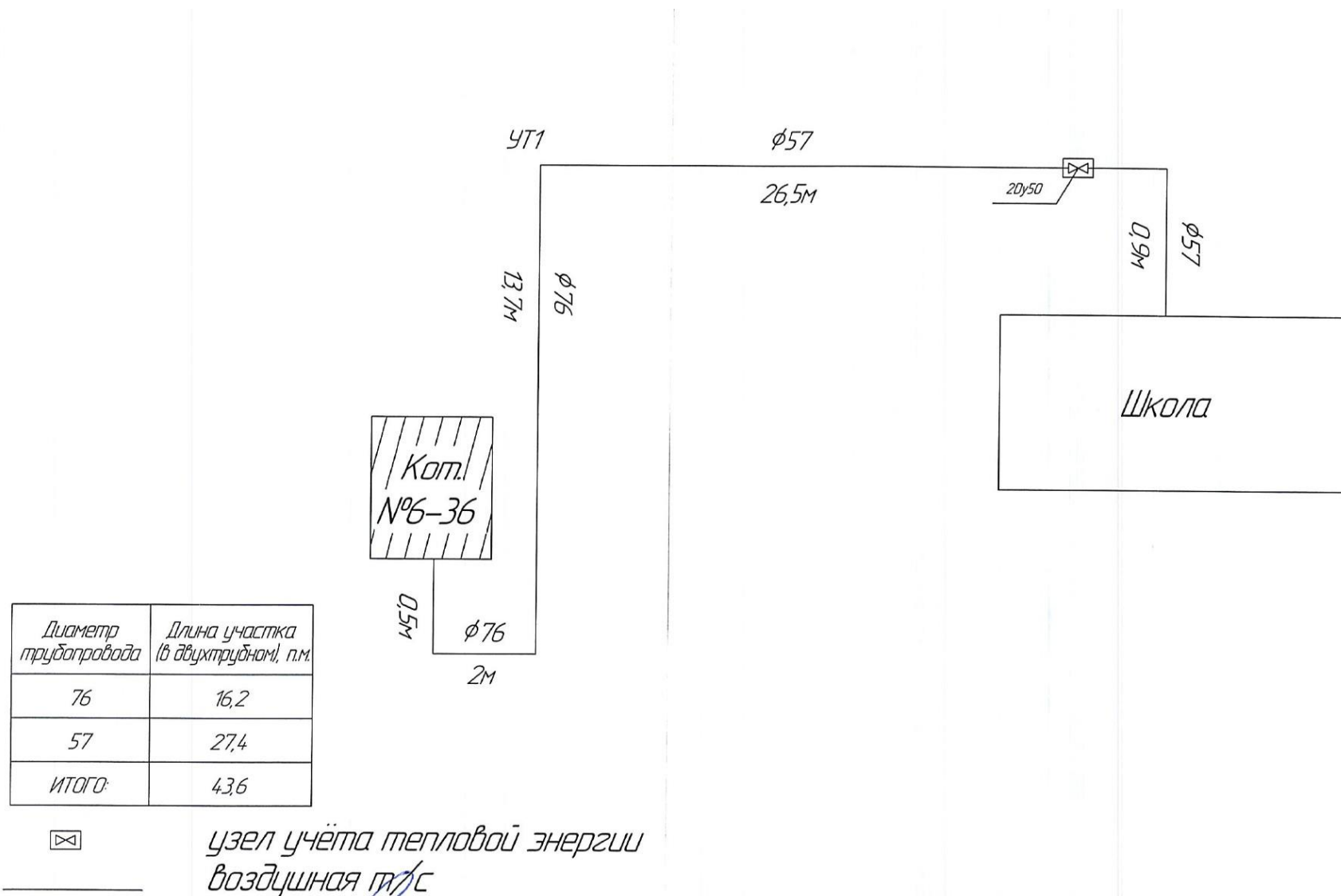
Рисунок 1.3.2.3 - Схема тепловых сетей котельной №6-36 с. Полудни
